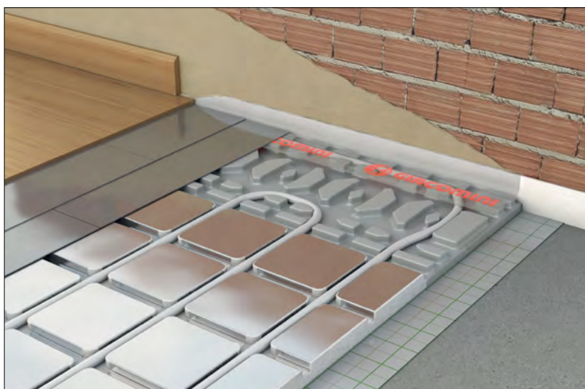
Příklad montáže s použitím R883-1 a R884 s krycími roznášecími plechy
