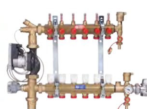
Rozdělovač R557FMS-W Varianty bez průtokoměrů nebo se skříni do zdi s čerpadlem Grundfos nebo Wilo
