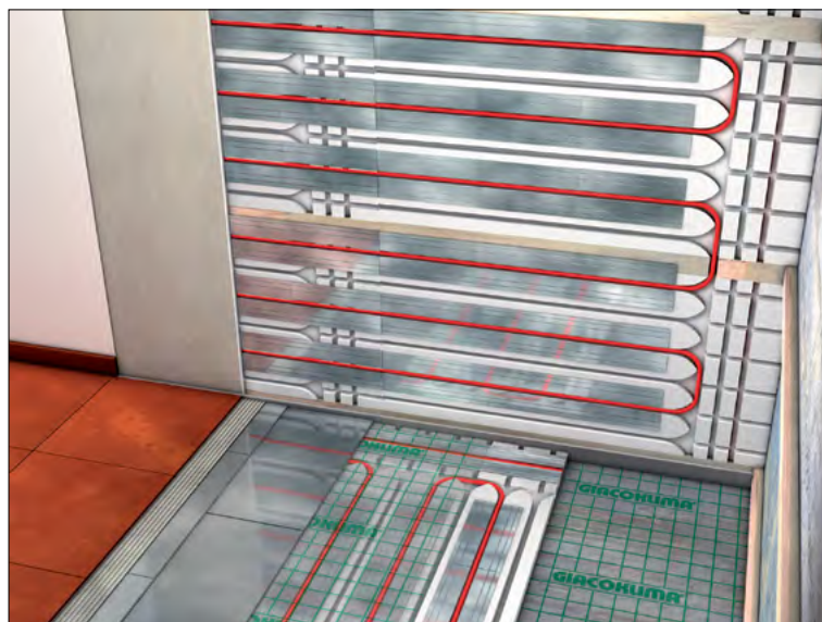
Příklad montáže stěnového a podlahového vytápění
