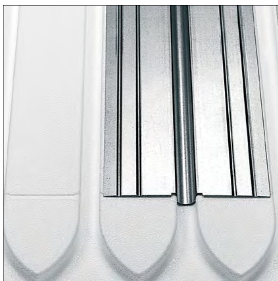
Systémová deska R883 s roznášecím plechem K802P
